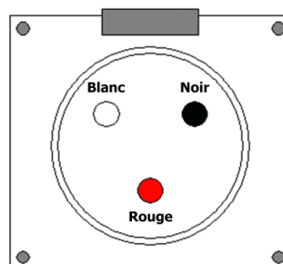
Prise femelle sur poste de pilotage Vue de dessus
